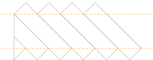
Abb. 13: Erste Reihe, mit Hilfslinien und Passstücken.
