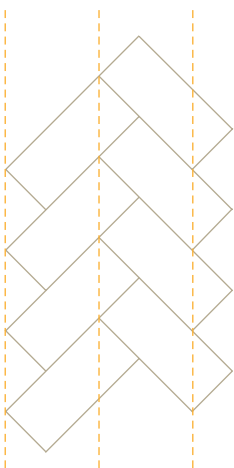
Abb. 5: Erste Reihe mit Hilfslinien.
