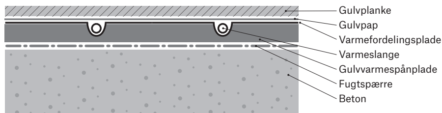
Figur 7: Længdesnit gulvvarmespånplade på beton
