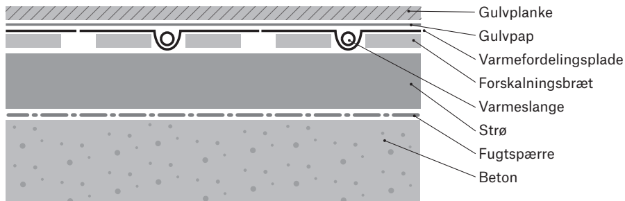
Figur 3: Tværsnit varmfedelingsplader på forskallingsbrædder oven på strøer
