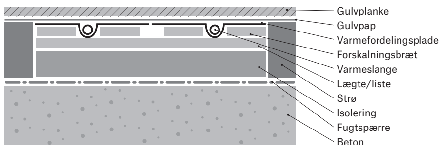
Figur 4: Længdesnit varmfedelingsplader på forskallingsbrædder mellem strøer
