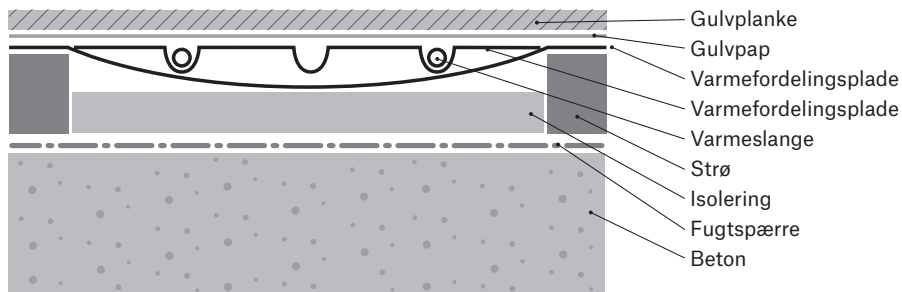
Figur 5: Længdesnit selv bærende varmfordelingsplader på strøer.
